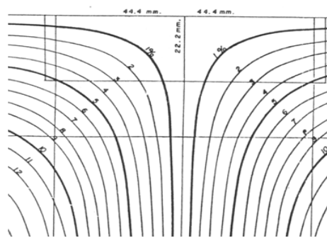
Figura 430.2.4 Curva ISO K de una luminaria simétrica para uso industrial
