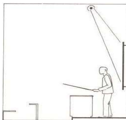
Figura 420.1.2 b. Alumbrado adicional sobre el tablero.
